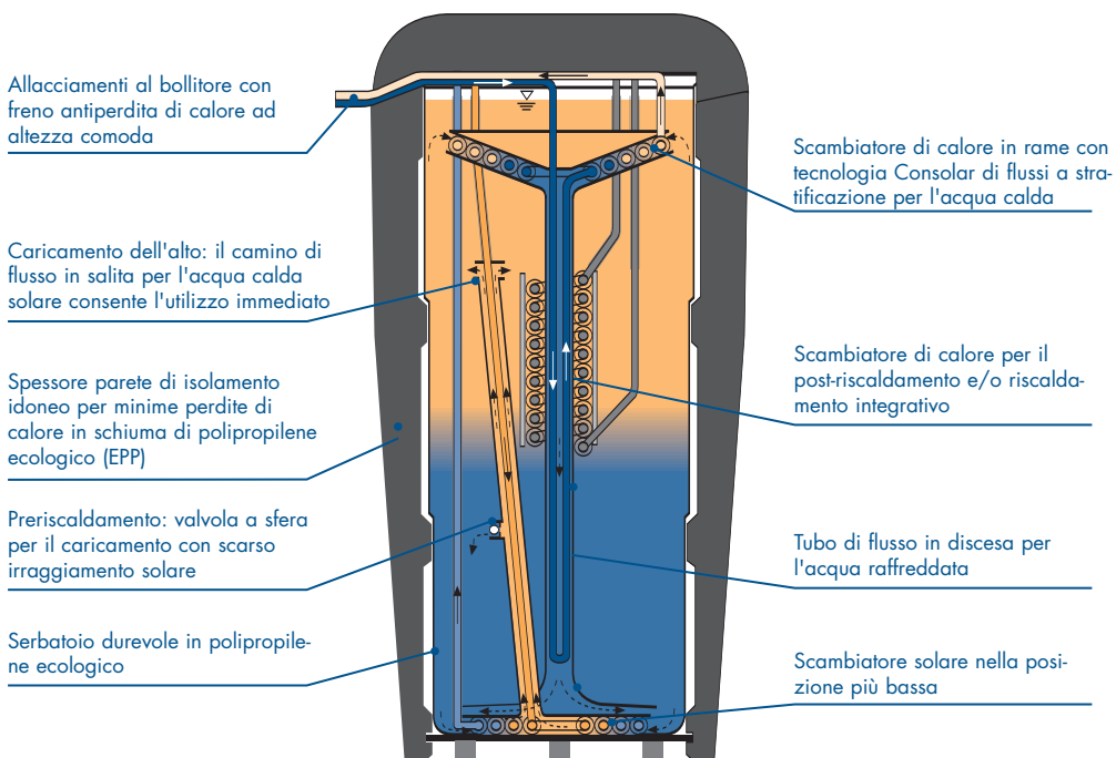
Sezione del CONUS 502
