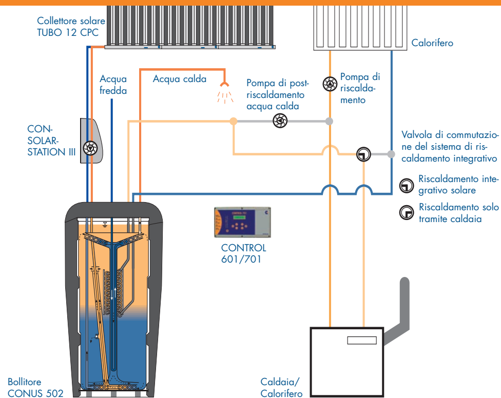
Schema tipico dell'installazione del CONUS 502 con aumento del ritorno per caldaia a gas e nafta
